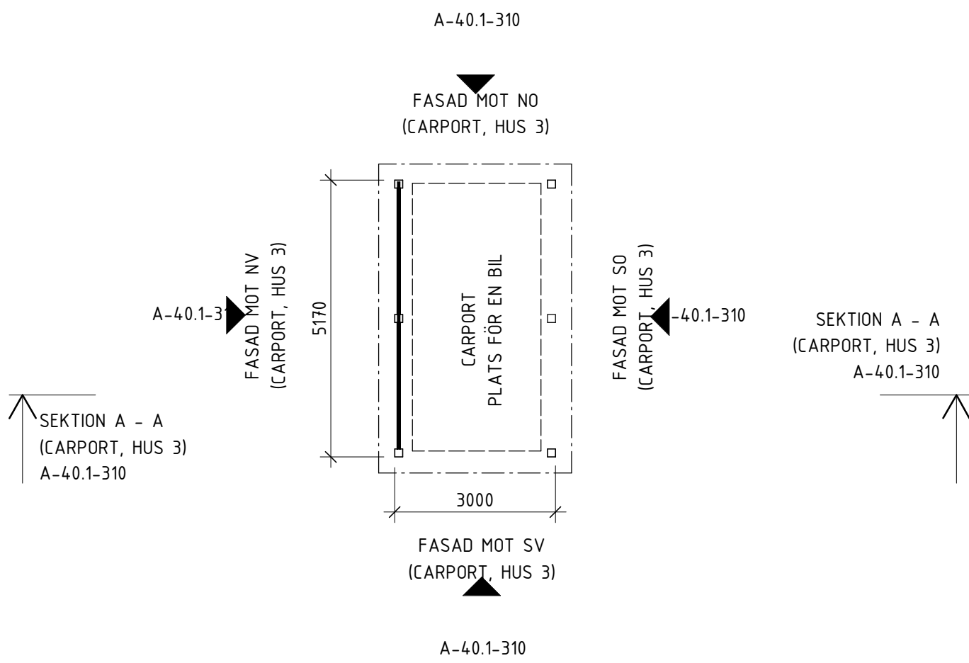
CARPORT - PLAN (HUS 3) 1 : 100
