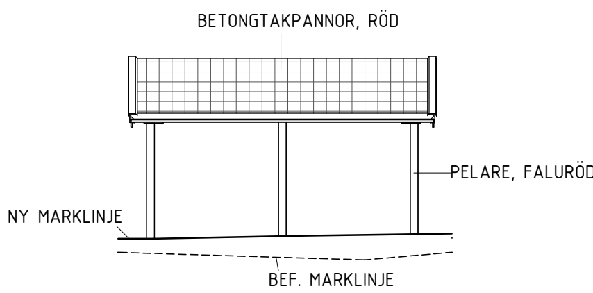
FASAD MOT SO (CARPORT, HUS 3) 1 : 100
