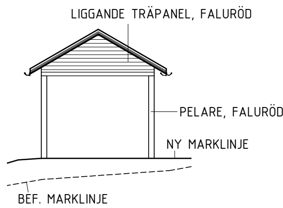
FASAD MOT SV (CARPORT, HUS 3) 1 : 100
