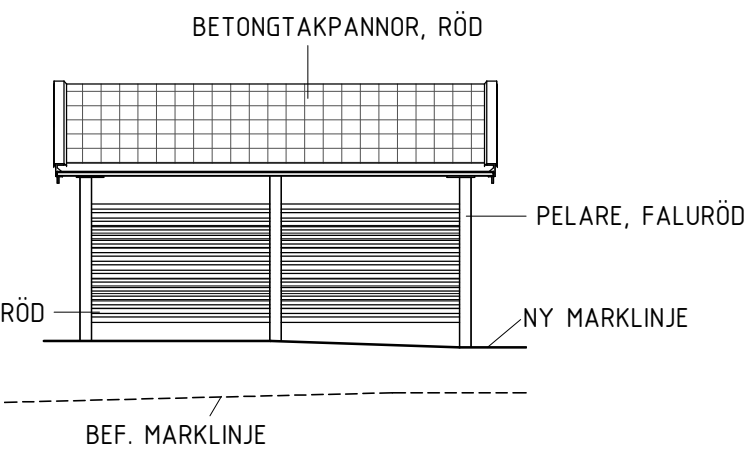
FASAD MOT NV (CARPORT, HUS 3) 1 : 100
