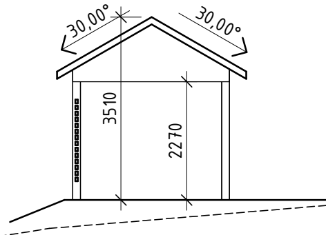
SEKTION A - A (CARPORT, HUS 3) 1 : 100
