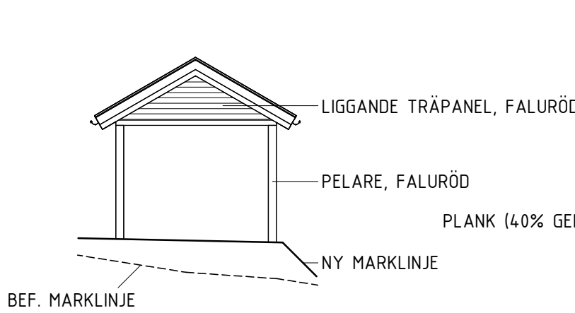
FASAD MOT NO (CARPORT, HUS 3) 1 : 100
